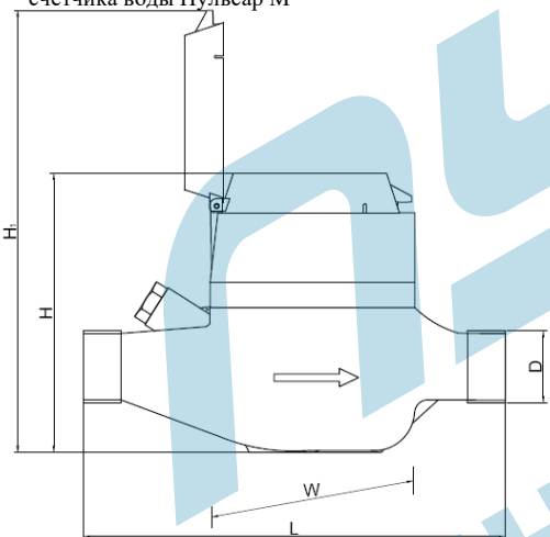
ПРИЛОЖЕНИЕ 1 Габаритные и присоединительные размеры счетчика воды Пульсар М
